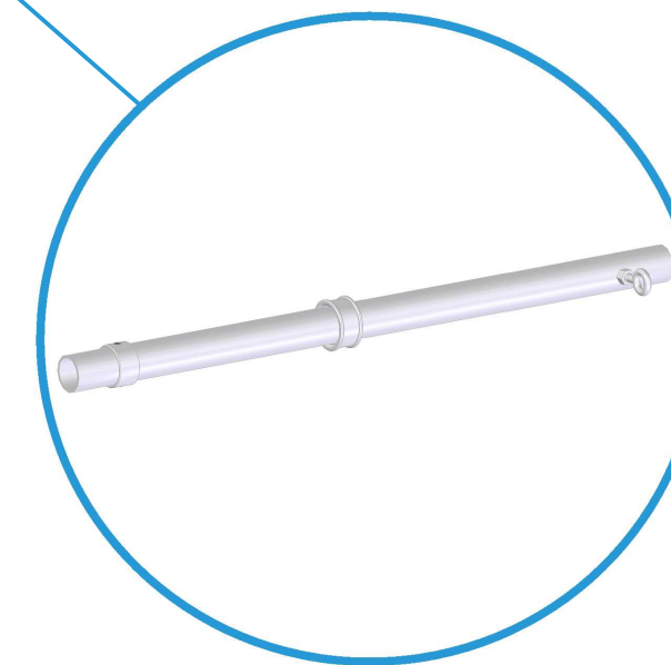
LISSE COULISSANTE Ø48,3x2,9 AVEC : - 1 BAGUE EN POLYAMIDE VISSEE - 1 BAGUE EN POLYAMIDE LIBRE - 1 ANNEAU DE FIXATION
