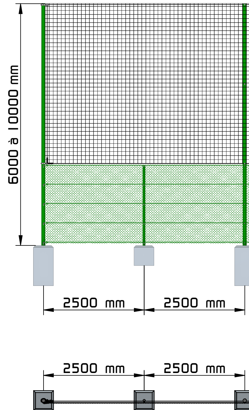
PARE BALLONS - GRILLAGE SIMPLE TORSION EN PARTIE BASSE
