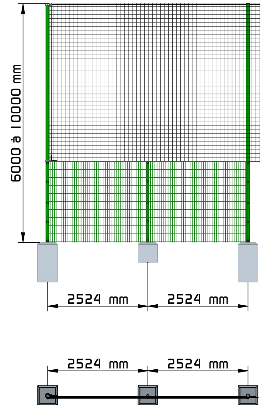
PARE BALLONS - PANNEAUX SOUDES EN PARTIE BASSE
